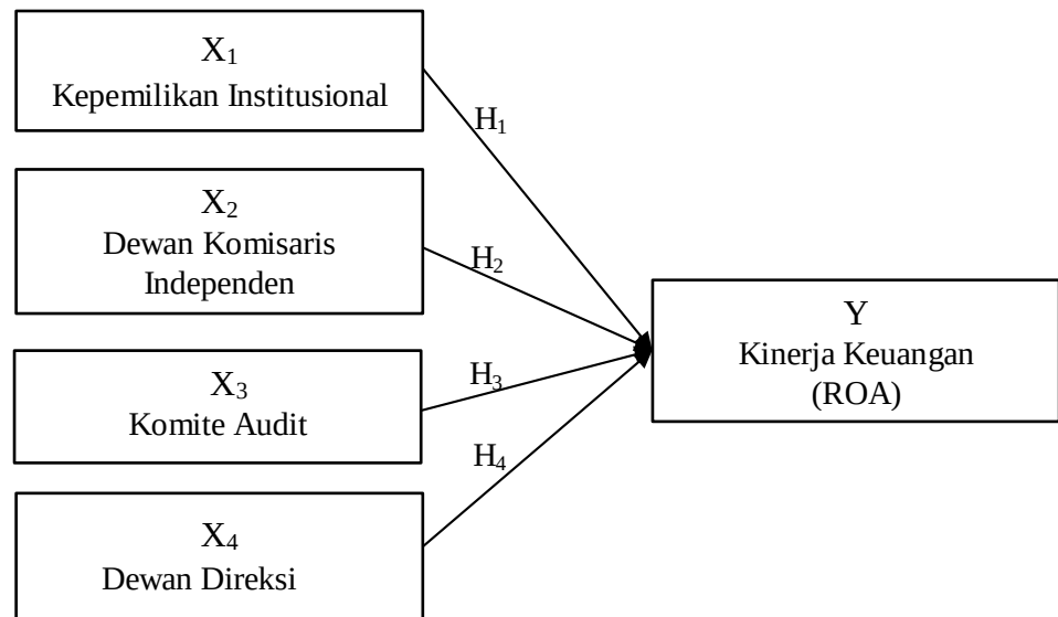
Gambar 1.1 Kerangka Pemikiran
